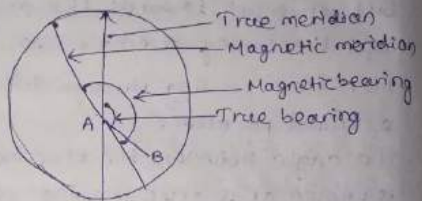
(Meridians)
